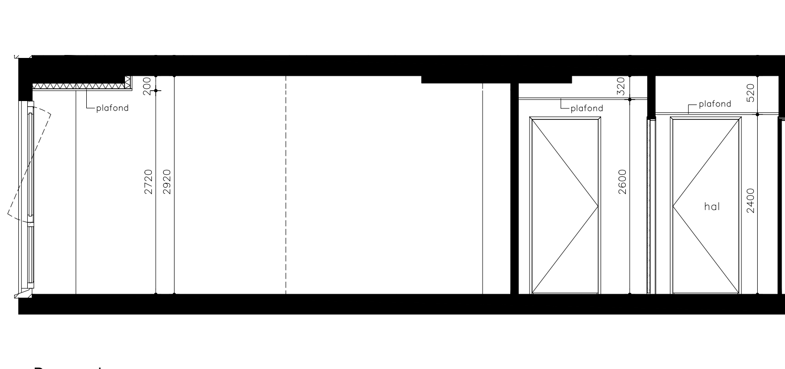
Doorsnede
