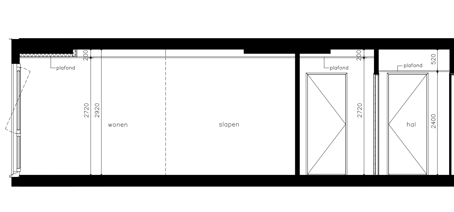
Doorsnede
